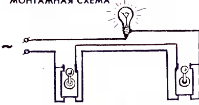
МОНТАЖНАЯ СХЕМА
